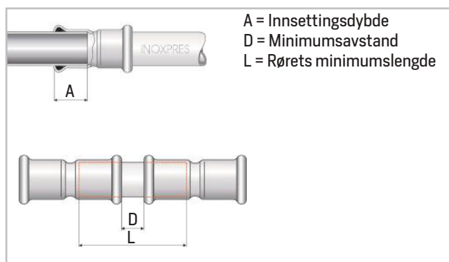
Bilde 27 - Innsettsdybde og minimumsavstander
